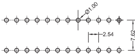
P.C.B. LAYOUT
