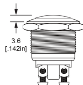
Domed Actuator
