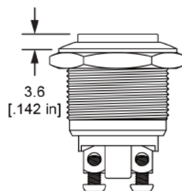
High Actuator
